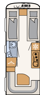
510 ER 4 Schlafplätze
