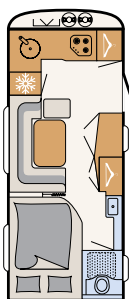
490 BLF
