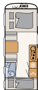
500 QSK 6 Schlafplätze
